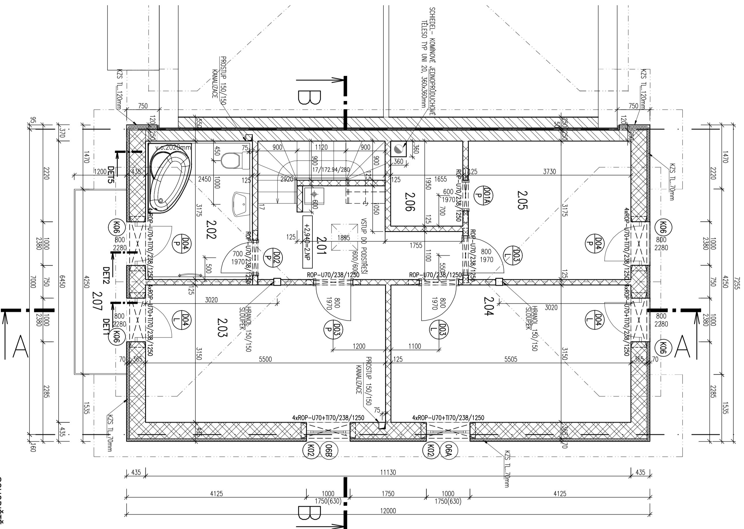
TABULKA MÍSTNOSTI
